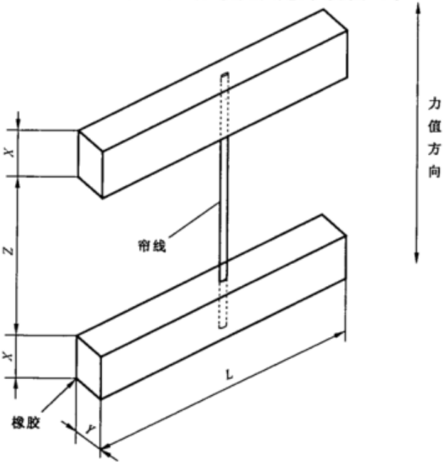
图 1 试样
