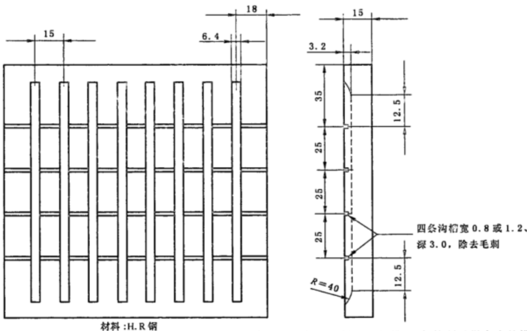
材料:H.R 钢
